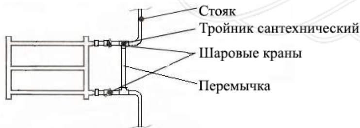
Рис.2 Шунтирующая обводка
