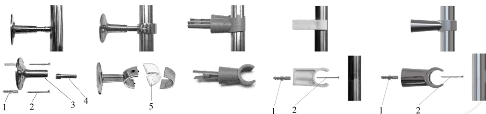
1-дюбель, 2-саморез, 3-опорная площадка, 4-шпилька, 5-прокладка
